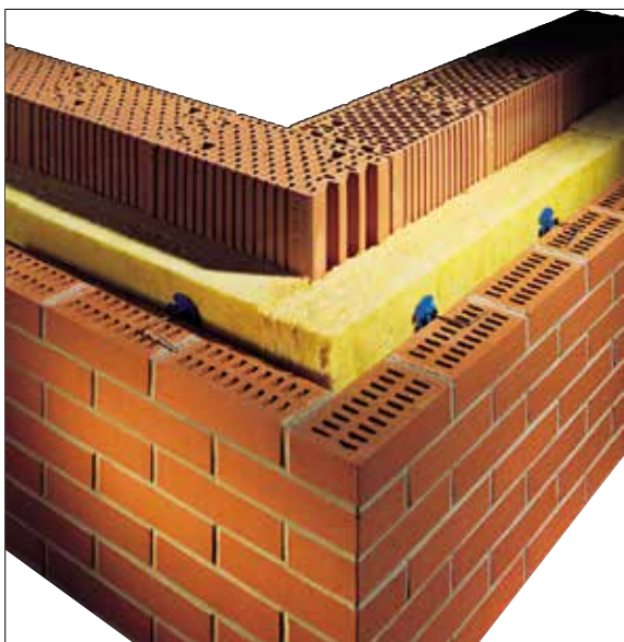
Trisluksnė siena
