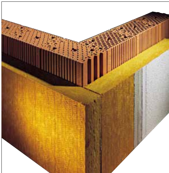
Dvisluksnė siena
